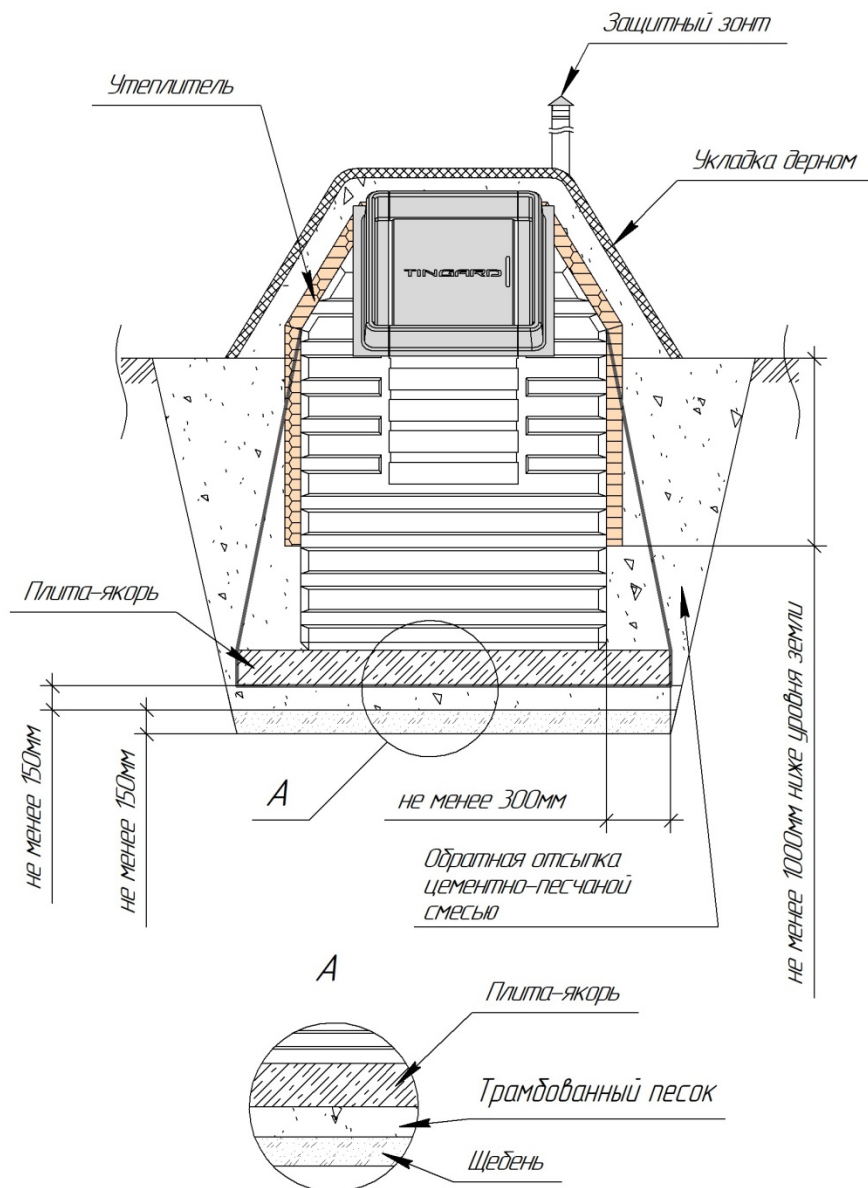
Схема монтажа погреба TINGARD 1900-Б, 2500-Б
