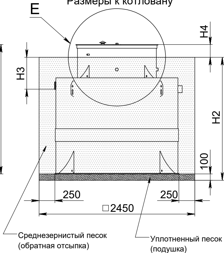
Размеры к котловану
