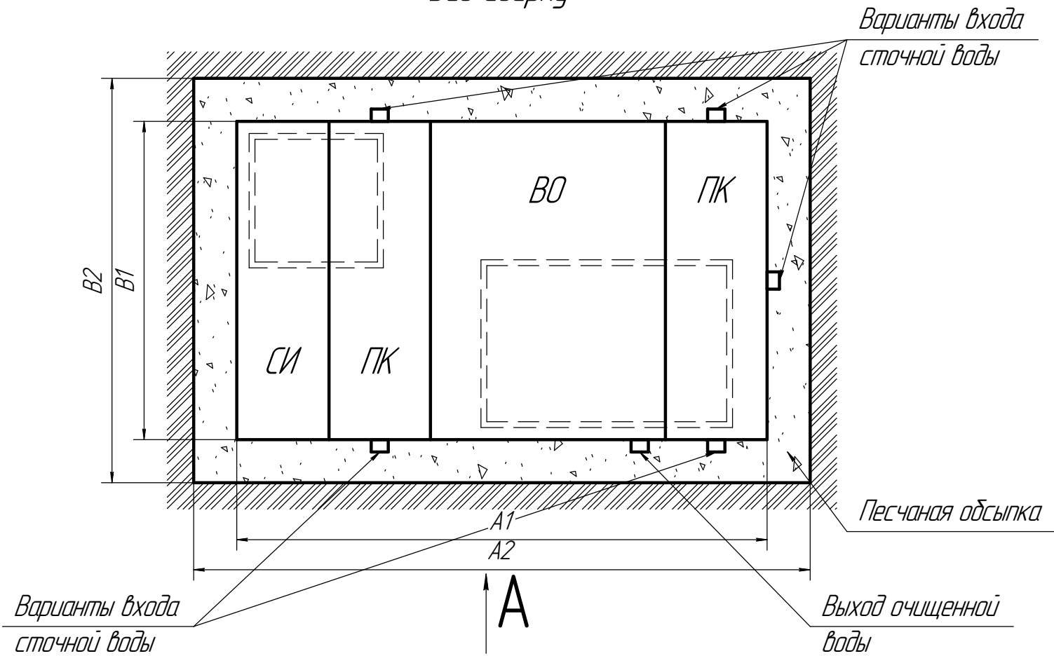
Вид сверху
