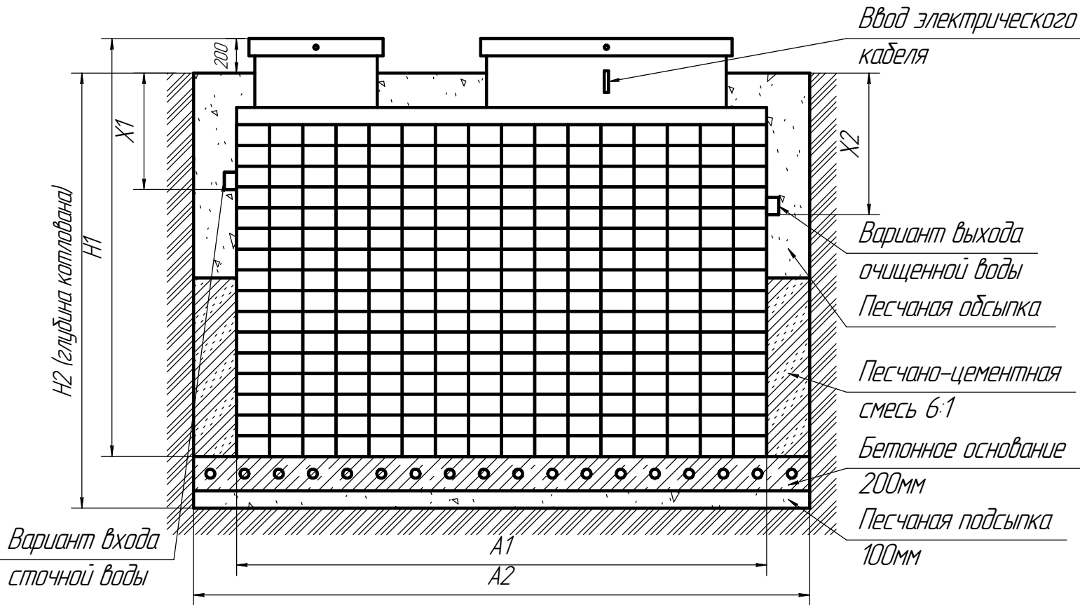
Вид А
