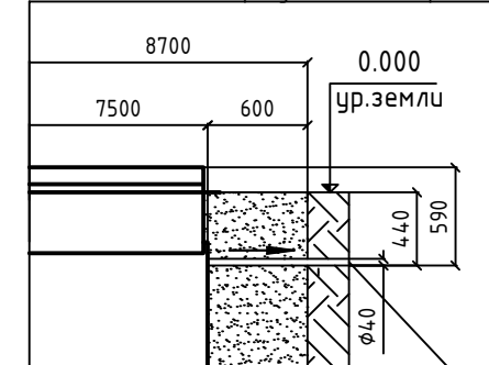
Вид А СХЕМА МОНТАЖА с принудительным сбросом
