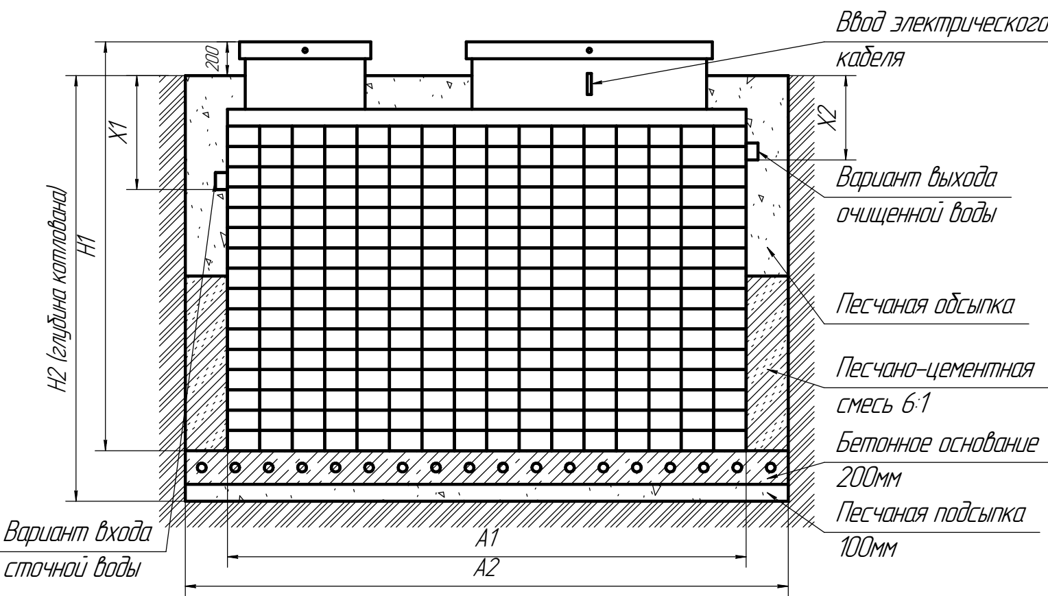
Вид А
