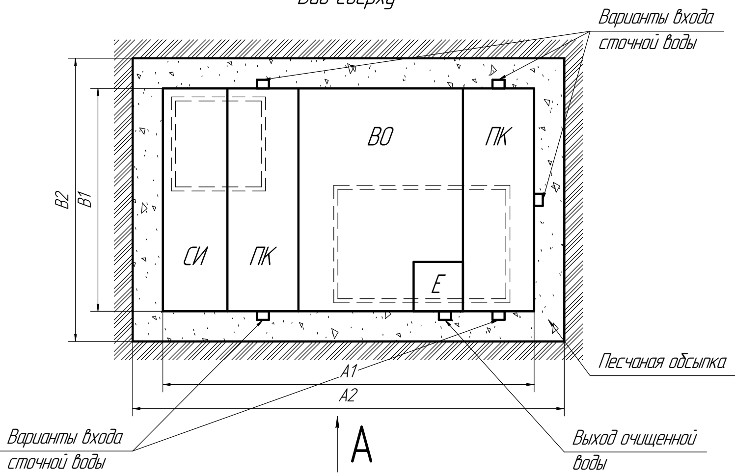
Вид сверху
